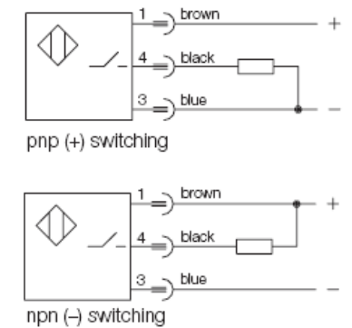
连接方式
